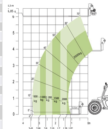
Rozsah pohybu ZTH2506E
