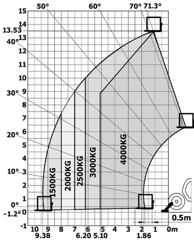
Diagram nosnosti MANITOU MT 1440
